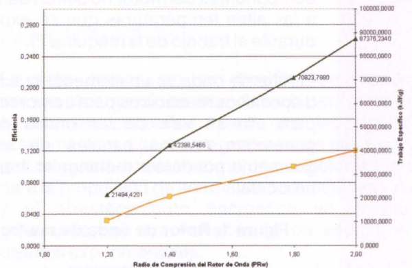
Figura 4. Eficiencia térmica y trabajo específico versus radio de presión del rotor de onda
