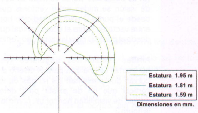
Fig. 2. Diagramas de alcance para la tripulación.
