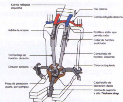
Fig. 9. Sistema de restricción modificado
